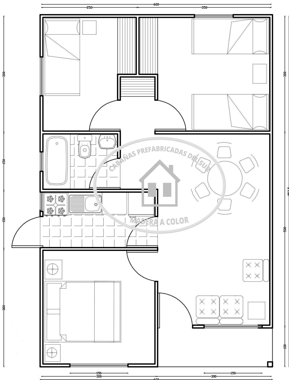
CABAÑA TIPO A 54 m2 (6 x 9)
