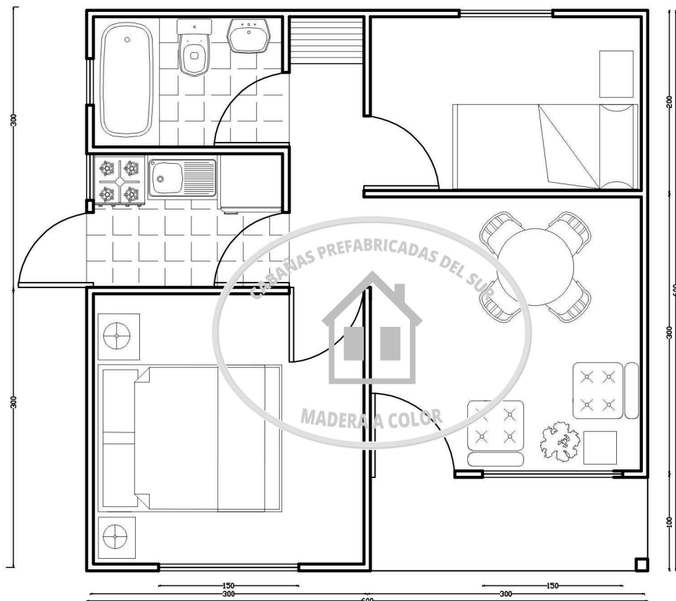
CABAÑA TIPO A 36 m2 (6 X 6)
