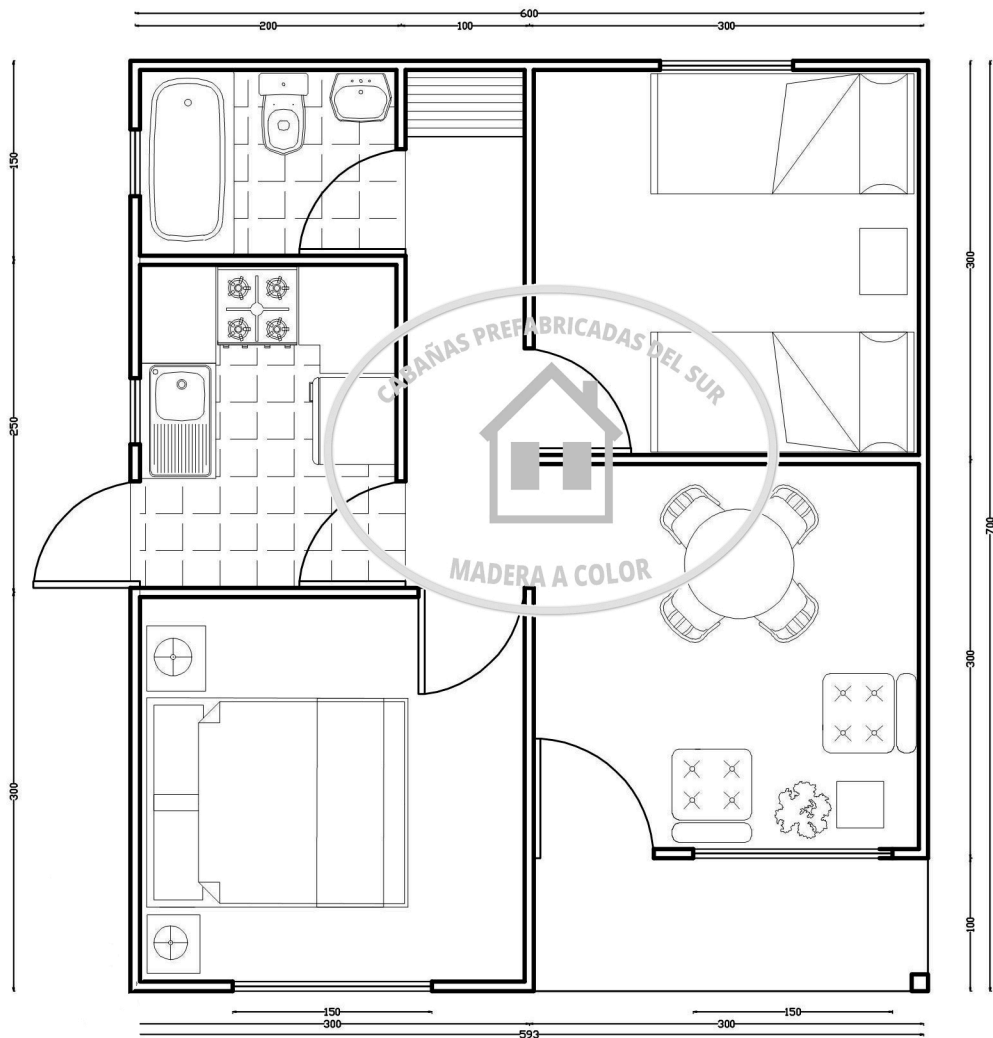
CABAÑA TIPO A 42 m2 (6 X 7)
